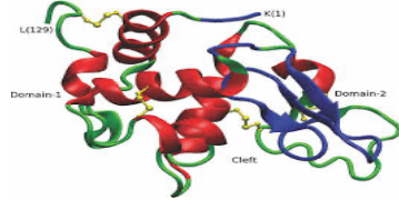
Lysozyme
